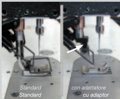
Adattatore del piedino di cucitura per gli organi di cucitura della PFAFF 938 Adaptor la picioruș pentru setul de coasere de la PFAFF 938
