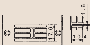
Placca-ago / Placa acului : 91-150 872-24/002
