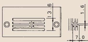
Placca-ago / Placa acului : 91-150 884-24/001
