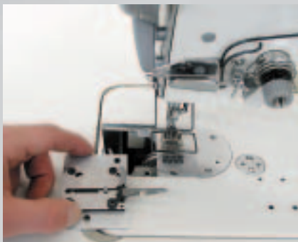
Dispositivo rasafio affidabile e sicuro -900/93
