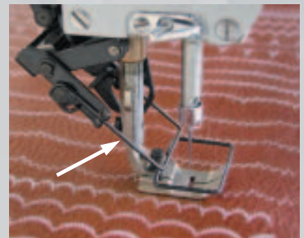
Dispositivo scartafilo -909/93 per un inizio cucitura pulito Retractor de fir -900/93 pentru un început de cusătură curat
