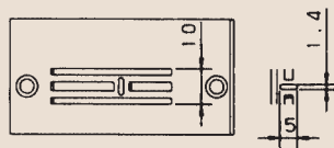
Placca-ago / Placa acului : 91-150 884-24/001
